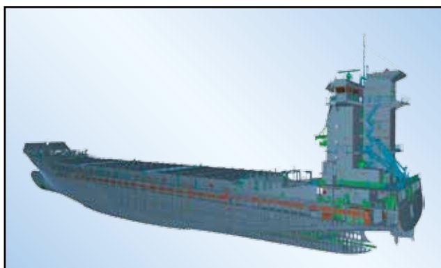
Модель контейнеровоза на 1036 TEU (20-футовых контейнеров), выполненная в системе Nupas-Cadmatic
