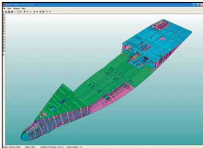
75-метровый сейнер/траулер, разработан компанией "Петронед" в системе Nupac-Cadmatic
