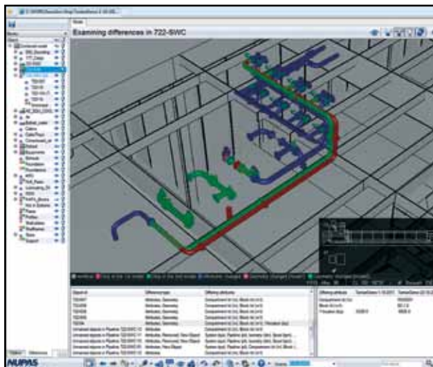
Легкое сравнение моделей в модуле eBrowser
