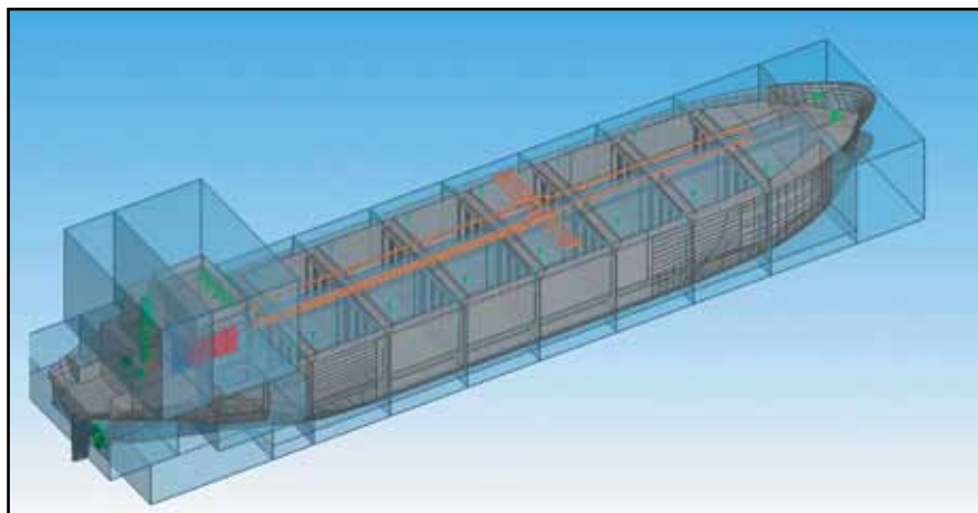
Использование отделений в Nupas-Cadmatic
